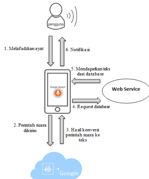
Gambar 4. Arsitektur dan alur kerja sistem
