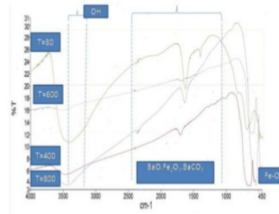
Gambar 3. Hasil pengujian tampa doping menggunakan FTIR dengan suhu 80, 400, 600 dan 800°C.
