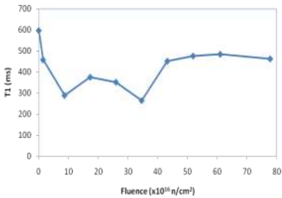
Gambar 4. Grafik waktu relaksasi spin-kisi (T1) metode pulsa 90 0 -τ-90 0 vs fluence neutron cuplikan polimer PVC.
