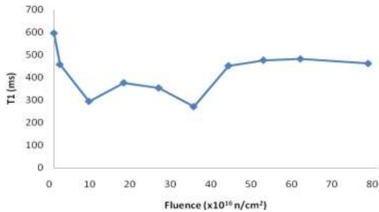
Gambar 3. Grafik waktu relaksasi spin-kisi (T1) metode pulsa 180 0 -τ-90 0 vs fluence neutron cuplikan polimer PVC.
