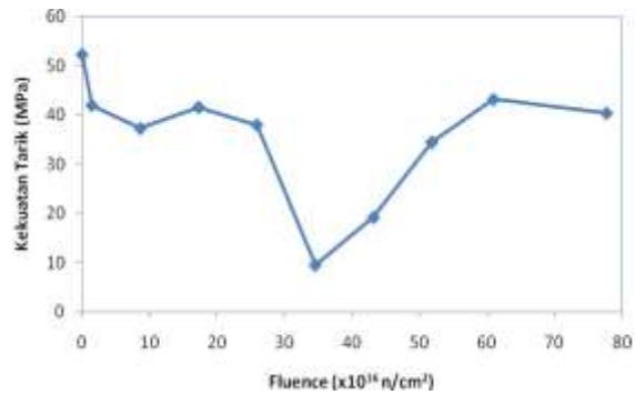
Gambar 5. Grafik kekuatan tarik vs fluence neutron cuplikan polimer PVC
