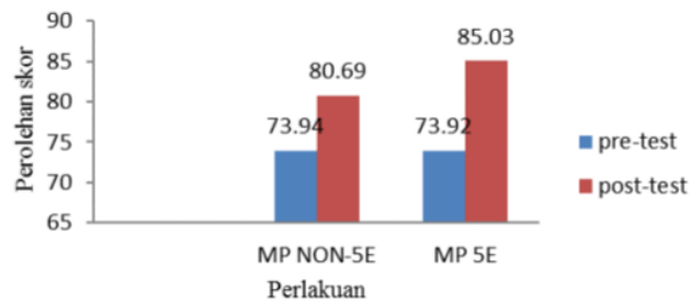
Gambar 2. Grafik perbandingan skor rata-rata sikap ilmiah peserta didik
