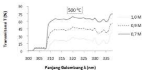
Gambar 3. Grafik spektrum transmitansi (T%) sebagai fungsi panjang gelombang ( \lambda )
