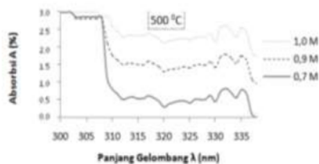
Gambar 4. Grafik spektrum absorptansi (A%) sebagai fungsi panjang gelombang ( \lambda )
