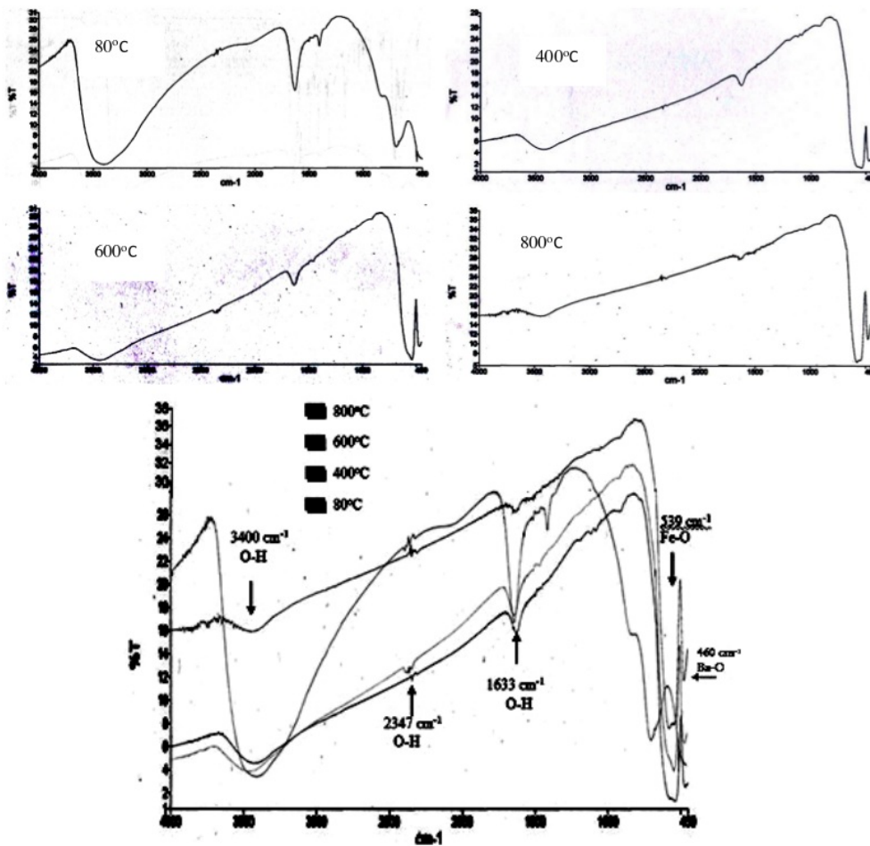
Gambar 3: Grafik pola penyerapan FTIR pada sampel \text{BaFe}_{12}\text{O}_{19} dengan variasi temperatur kalsinasi.
