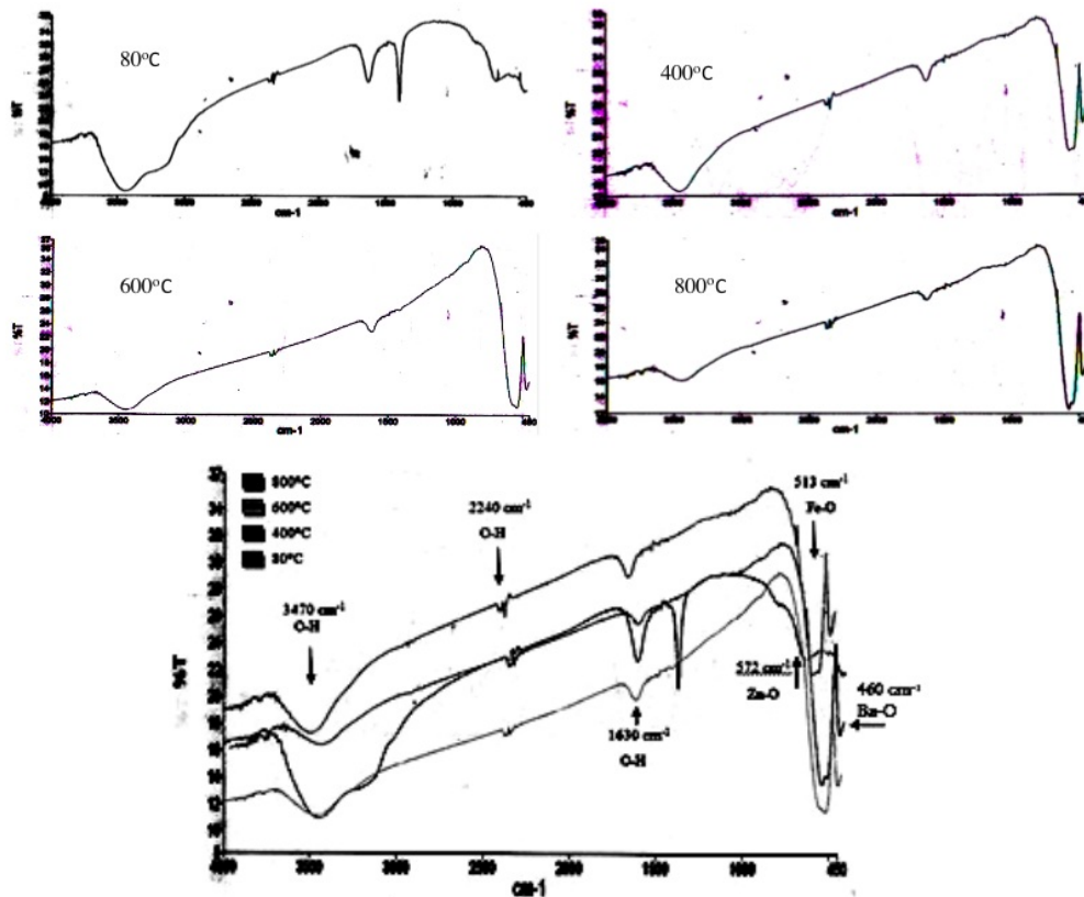
Gambar 5: Grafik pola penyerapan FTIR pada sampel BaFe 11.4 Zn 0.6 O 19 dengan variasi temperatur kalsinasi
