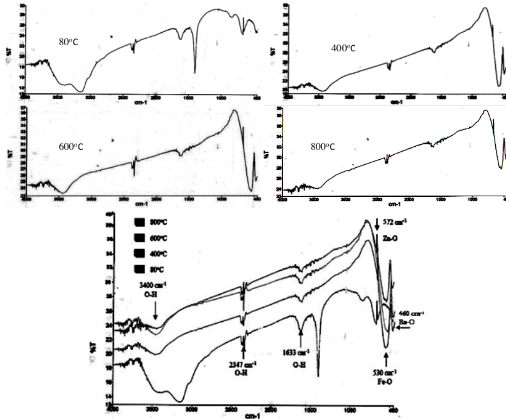
Gambar 4: Grafik pola penyerapan FTIR pada sampel BaFe 11,7 Zn 0,3 O 19 dengan variasi temperatur kalsinasi.
