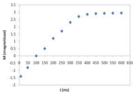
Gambar 1. Grafik hubungan amplitudo sinyal peluruhan magnetisasi (M) sebagai fungsi waktu (t) hasil pengukuran penentuan waktu relaksasi (T1) metode pulsa 180^0\text{-}\tau\text{-}90^0
