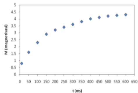
Gambar 2. Grafik hubungan amplitudo sinyal peluruhan magnetisasi (M) sebagai fungsi waktu (t) hasil pengukuran penentuan waktu relaksasi (T1) metode pulsa 90^0\text{-}\tau\text{-}90^0
