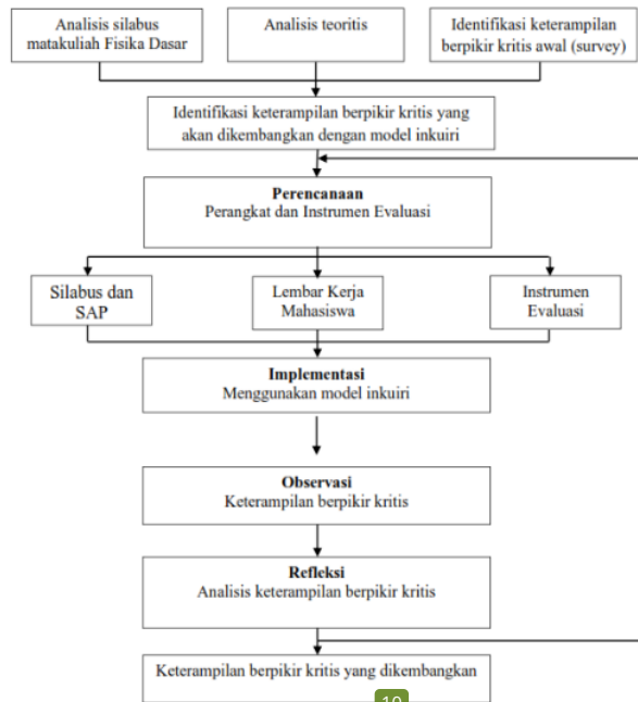
Gambar 1. Desain Penelitian
