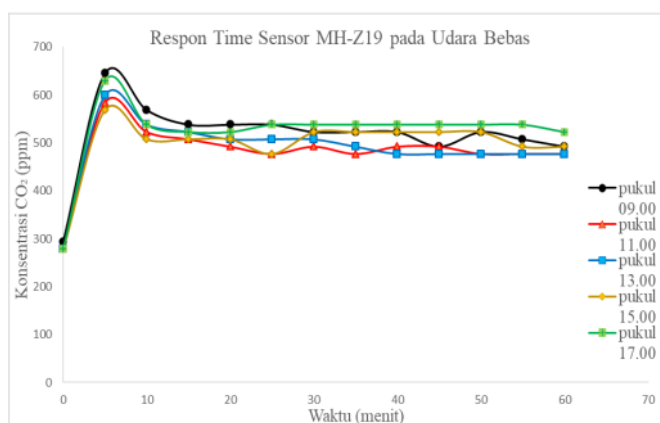
Gambar 3. Response Time Sensor Terhadap Udara Bebas.
