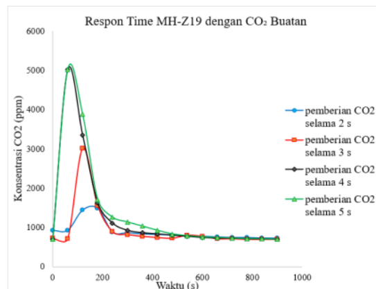
Gambar 5. Response time pemberian CO 2 buatan.
