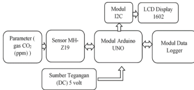
Gambar 1. Diagram Blok Sistem Pendeteksi Penyerapan CO 2 .
