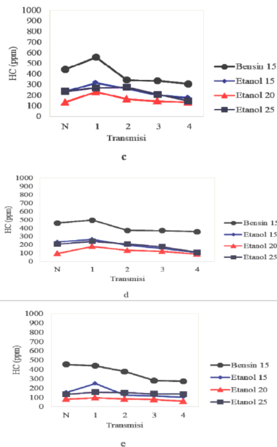
Gambar 6. Hubungan emisi gas buang HC pada tingkat transmisi dan waktu pembakaran; (a) 1500 rpm, (b) 2500 rpm, (c) 3500 rpm, (d) 4500 rpm, dan (e) 6000 rpm
