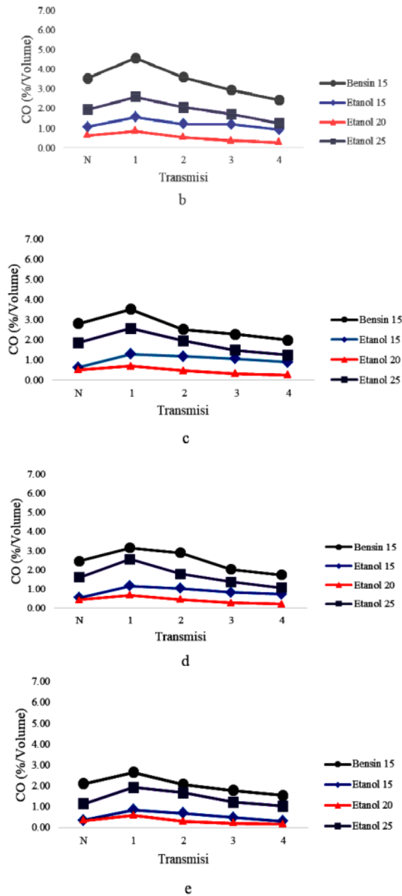
Gambar 4. Hubungan emisi gas CO dengan tingkat transmisi dan waktu pembakaran; (a) 1500 rpm, (b) 2500 rpm, (c) 3500 rpm, (d) 4500 rpm, (e) 6000 rpm.
