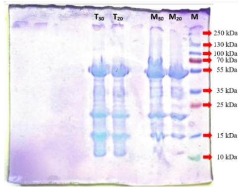
Gambar 1. Gel hasil elektroforesis marker dan sampel
