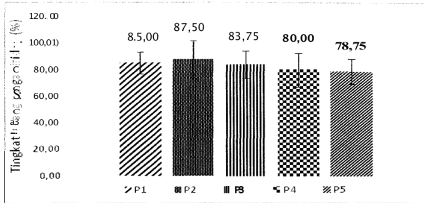
Gambar 1. Tingkat kelangsungan hidup ikan bawal bintang ( T. blochii ) dengan debit air yang berbeda pada saat pergantian air
