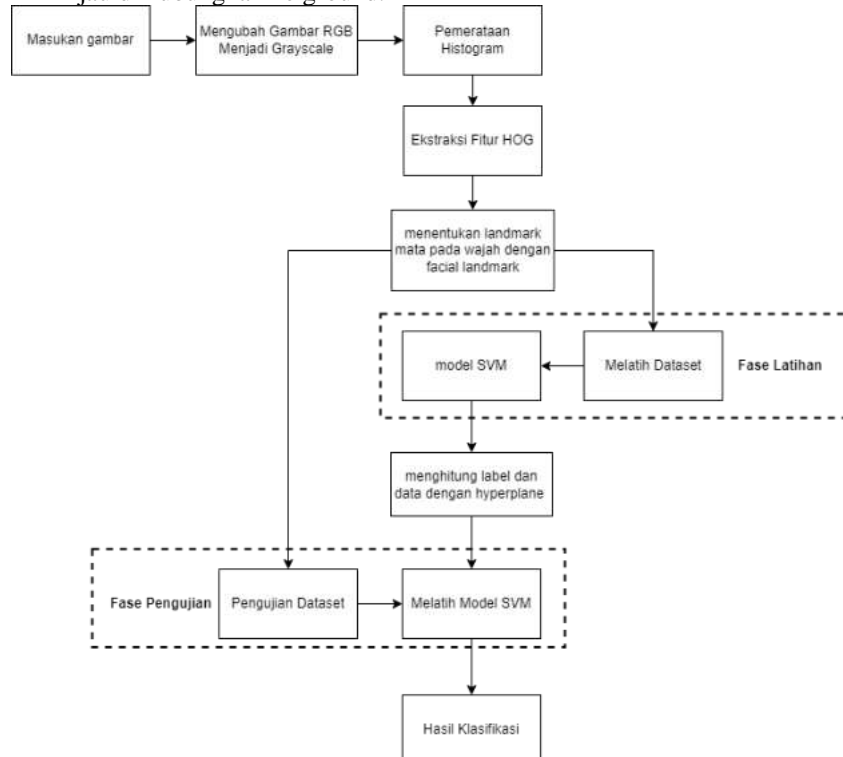
Gambar 7 Blok Diagram Algoritma HOG+SVM
