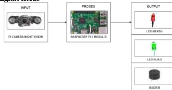
Gambar 10 Blok Diagram Perangkat Keras
