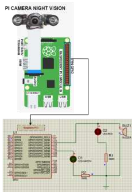
Gambar 6 Perancangan Alat Pendeteksi kantuk
