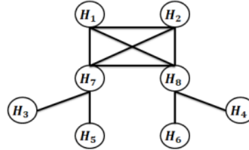
Gambar 3.2 Graf irisan D_{2,4}
