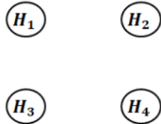
Gambar 3.1 Graf irisan dari D_{2,3}
