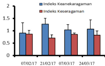
Gambar 7. Rata-rata indeks keaneekaragaman dan keseragaman spesies Dinophyta antar waktu penelitian. Batang galat menunjukkan standar deviasi.
