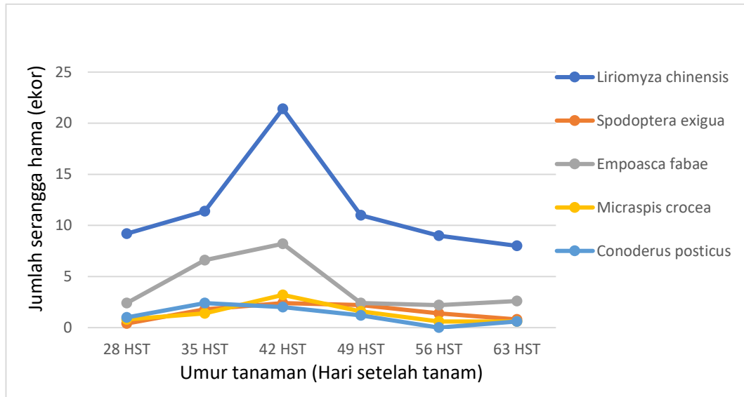
Gambar 1. Perkembangan populasi serangga hama umur 28 HST-63 HST
