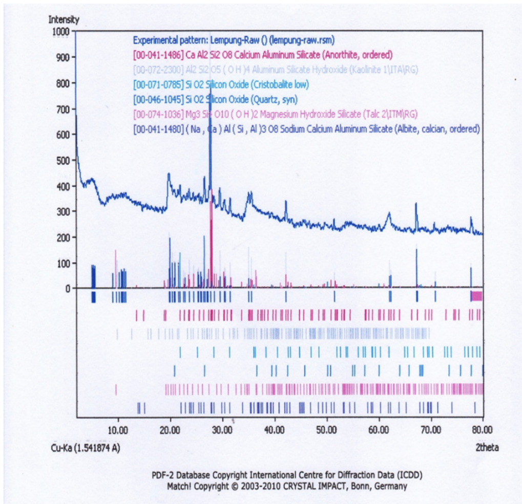
Gambar 5. Hasil uji XRD tanah lempung
