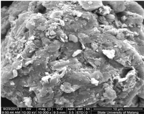
Gambar 6. Hasil uji SEM tanah lempung pembesaran 10.000 kali
