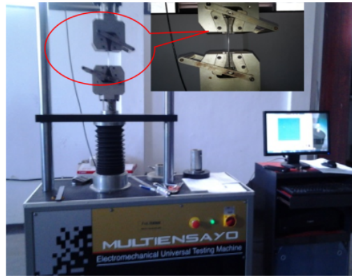
Gambar 7. Foto uji kuat tarik plastik
