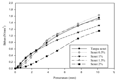
Gambar 13. Grafik hubungan antara Beban dengan penurunan (panjang serat=25mm)
