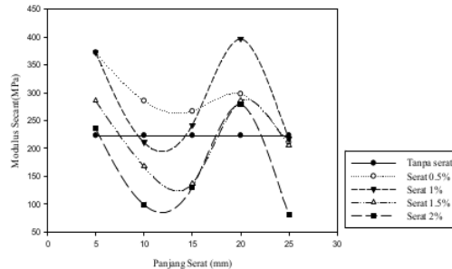
Gambar 15. Grafik hubungan nilai modulus secant dengan panjang dan prosentase serat
