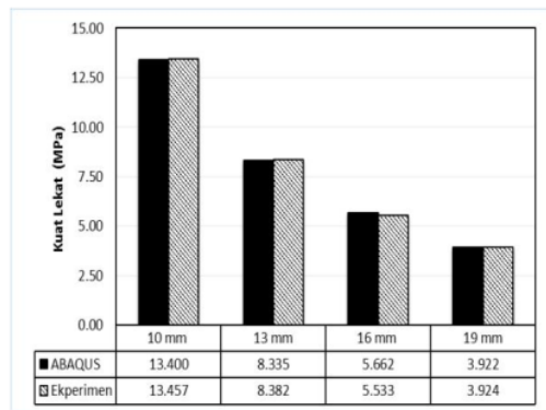
Gambar 11. Perbandingan kuat lekat eksperimen dan pemodelan
