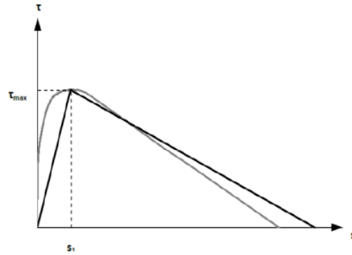
Gambar 3. Pendekatan dari hubungan lekatan-slip eksperimen (garis abu) dengan hukum traction separation (garis hitam) (Molina et al., 2015)
