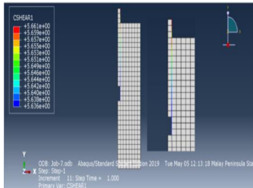
Gambar 9. Kuat lekat yang terjadi pada tulangan diameter 16 mm
