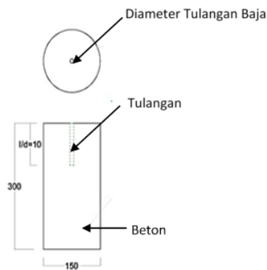
Gambar 5. Benda uji eksperimen (Wulandari, 2019)
