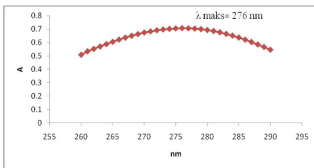
Gambar 1. Grafik panjang gelombang maksimum
