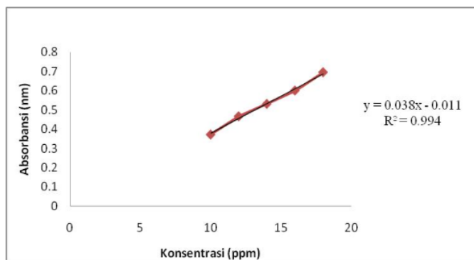
Gambar 2. Grafik kurva baku natrium diklofenak
