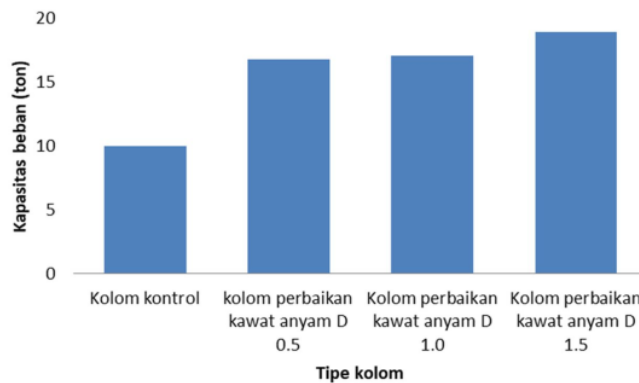
Gambar 5. Kapasitas Beban Kolom
