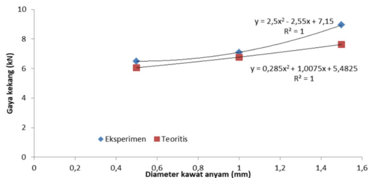
Gambar 6. Efek Pengekangan Secara Teoritis
