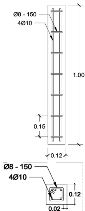
Gambar 2. Dimensi dan Detail Penulangan Kolom
