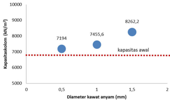
Gambar 7. Kapasitas Kolom per Satuan Luas Penampang
