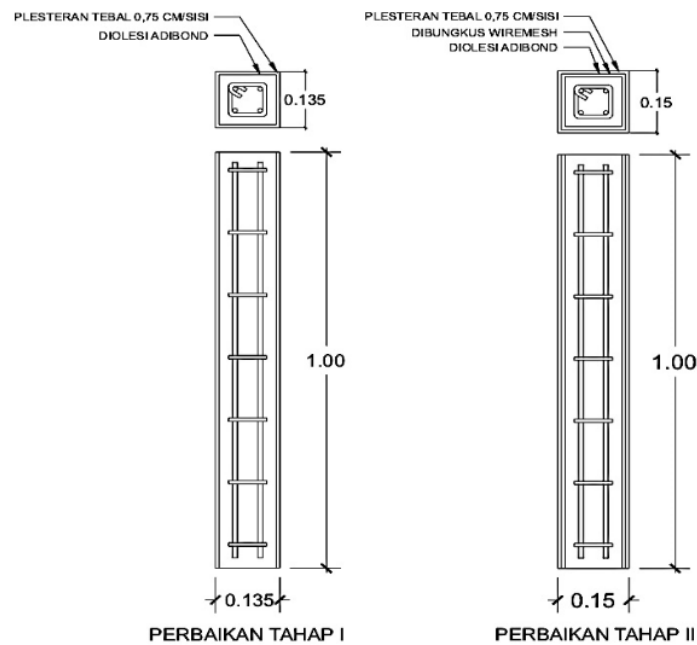
Gambar 4. Detail Perbaikan Kolom
