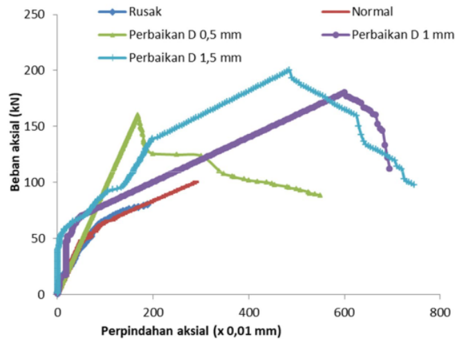
Gambar 9. Hubungan Antara Beban Dan Perpindahan Aksial
