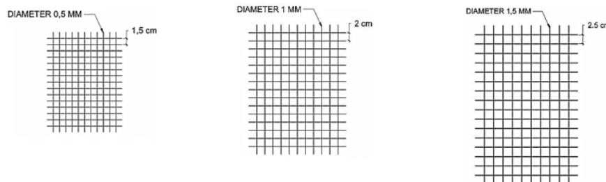
Gambar 1. Variasi Kawat Anyam
