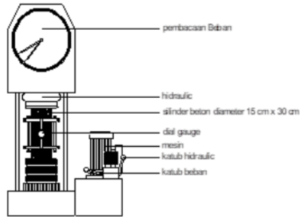
Gambar 4. Setting up uji kuat tekan
