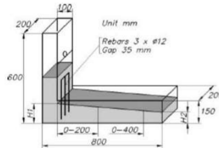
Gambar 3. L-box Test (EFNARC, 2005)
