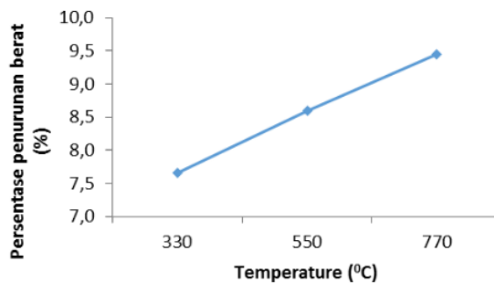
Gambar 2 Penurunan Berat Beton Pasca Bakar
