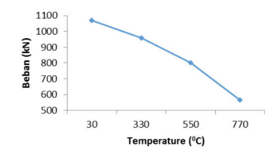
Gambar 3 Penurunan Kapasitas Beban Tekan Beton Pasca Bakar
