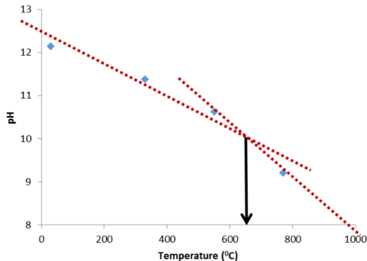
Gambar 5. Onset Temperatur Peralihan Asam-Basa Beton Pasca bakar
