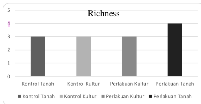
GAMBAR 3 Tingkat kekayaan spesies ( species richness )
