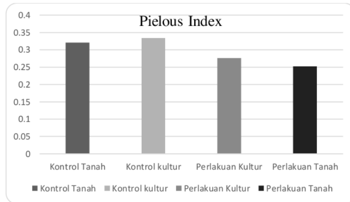
GAMBAR 5 Indeks Kemerataan Pielous
