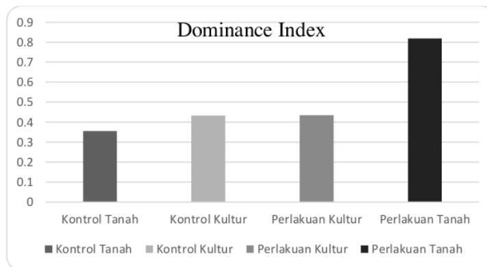
GAMBAR 6 Indeks Dominansi Simpson
