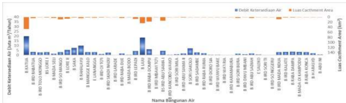
Gambar 7. Debit Ketersediaan air terhadap Luas Cacthment Area pada Bangunan Air yang berada di Daerah Aliran Sungai (DAS) Rabalaju Wilayah Sungai (WS) Sumbawa
