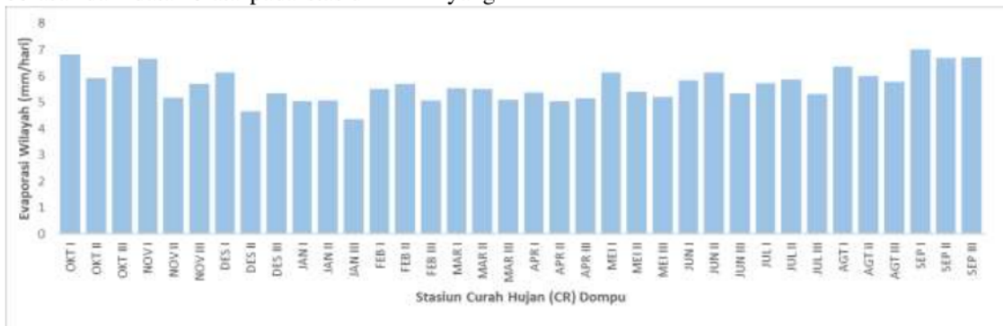
Gambar 5. Nilai Evaporasi pada stasiun iklim (CR) Dompu di Daerah Aliran Sungai (DAS) Rabalaju Wilayah Sungai (WS) Sumbawa
