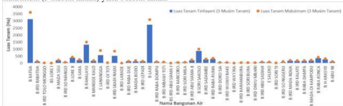
Gambar 9. Luas tanam yang terlayani pada Bangunan Air yang berada di Daerah Aliran Sungai (DAS) Rabalaju Wilayah Sungai (WS) Sumbawa.
