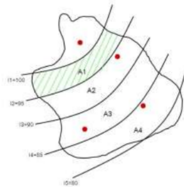
Gambar 1. Ilustrasi Metode Isohyet dimana terdapat 4 Stasiun hujan (ARR)
