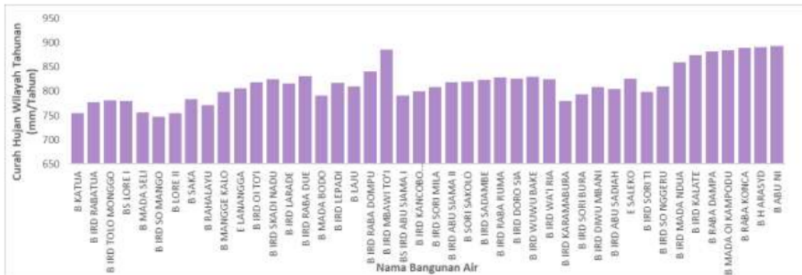
Gambar 4. Nilai Curah Hujan pada stasiun Curah Hujan (ARR) Dompu di Daerah Aliran Sungai (DAS) Rabalaju Wilayah Sungai (WS) Sumbawa
