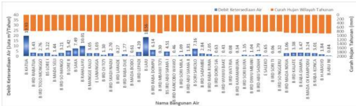
Gambar 6. Debit Ketersediaan air terhadap curah hujan tahunan pada Bangunan Air yang berada di Daerah Aliran Sungai (DAS) Rabalaju Wilayah Sungai (WS) Sumbawa
