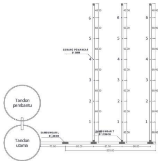
Gambar 1 Sketsa jaringan irigasi perforasi tampak atas
