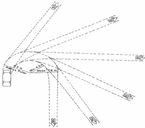
Gambar 3. Jari-jari Manuver Mobil Penumpang
