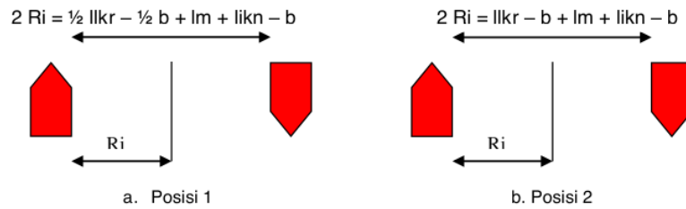
Gambar 10. Sketsa besarnya R_i
