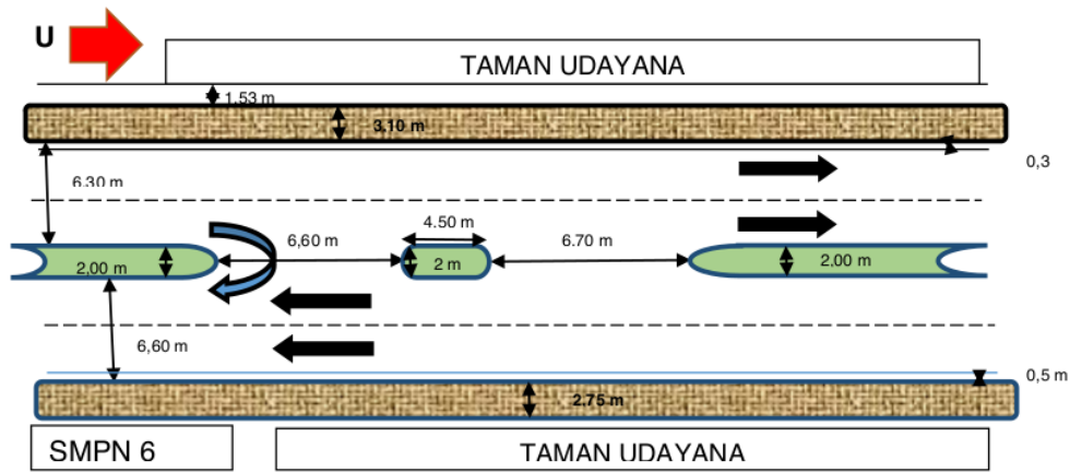
Gambar 6. Sketsa lokasi di ruas jalan Udayana
