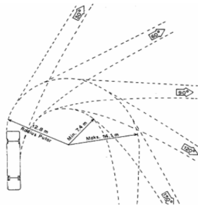
Gambar 4. Jari-jari Manuver Kendaraan Sedang
