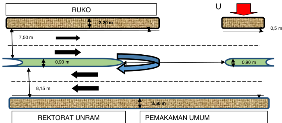
Gambar 7. Sketsa lokasi di ruas jalan Majapahit I
