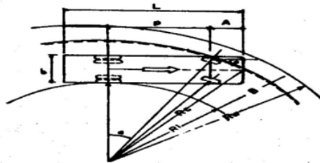
Gambar 5. Kondisi pada saat off tracking
