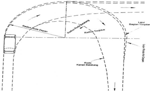
Gambar 2. Jari-jari Manuver Kendaraan
