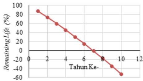
Gambar 6. Penurunan Umur Rencana pada Muatan Berlebih
