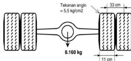
Gambar 2. Sumbu Standar 8.16 ton
