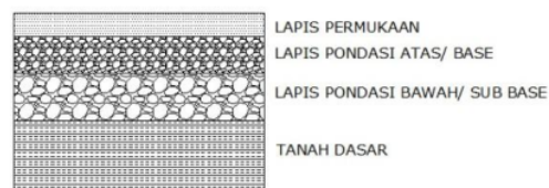
Gambar 1. Lapisan Perkerasan Lentur (Sumber: Sukirman, 2010)
