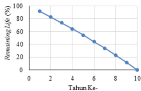
Gambar 5. Penurunan Umur Rencana pada Muatan Normal
