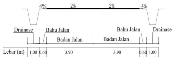
Gambar 4. Potongan Melintang Jalan Ahmad Yani.
