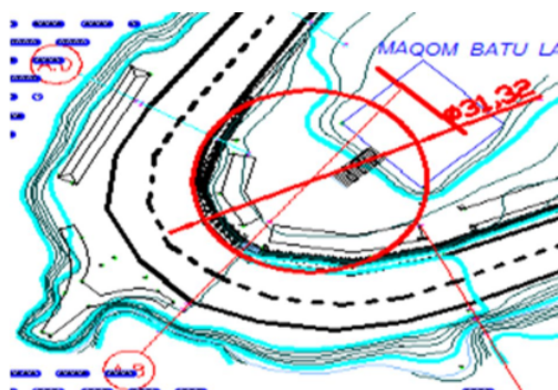
Gambar 2. Hasil ukur diameter tikungan Batu Layar
