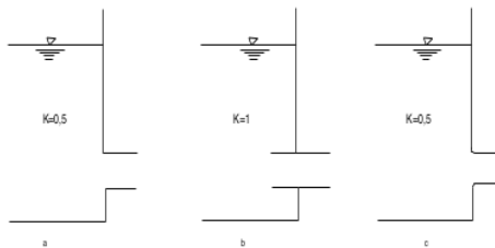
Gambar 1. Bentuk bentuk lubang pemasukan pipa
