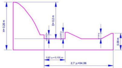
Gambar 3. Rancangan bendung
