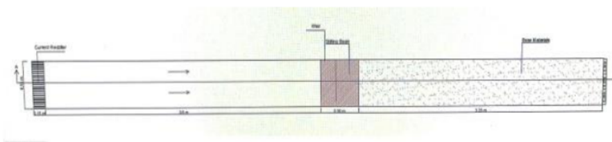
Gambar 2. Rancangan penempatan bendung pada saluran
