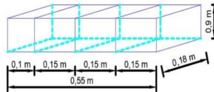
Gambar 4. Rancangan bronjong
