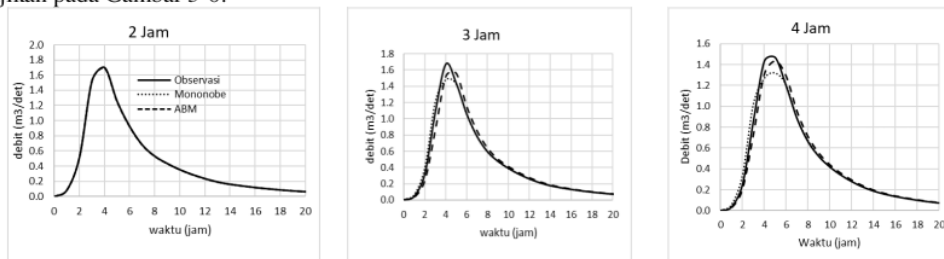
Gambar 3. Hidrograf banjir untuk distribusi hujan 2, 3 dan 4 jam
