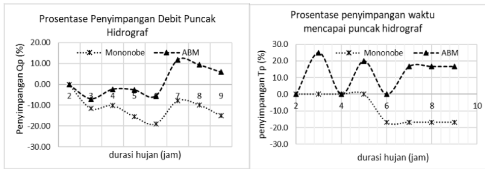
Gambar 6. Prosentase penyimpangan Qp dan Tp
