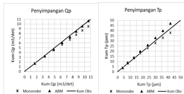
Gambar 6. Penyimpangan nilai Qp dan Tp
