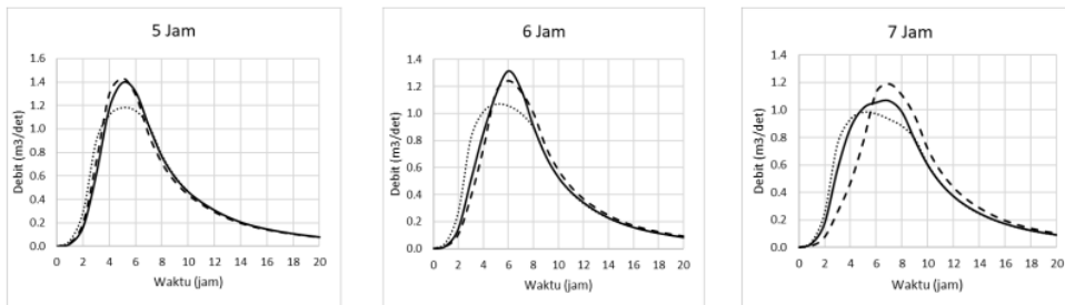
Gambar 4. Hidrograf banjir untuk distribusi hujan 5,6, dan 7 jam
