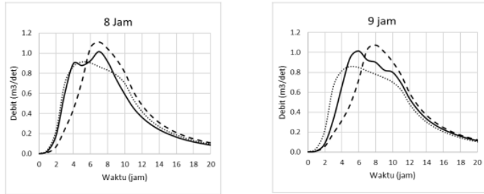
Gambar 5. Hidrograf banjir untuk distribusi hujan 8 dan 9 jam
