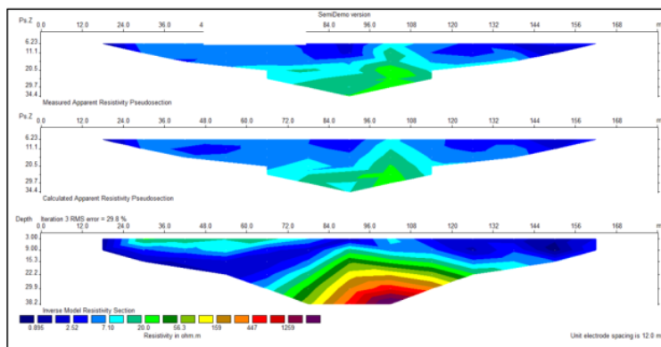
Gambar 6 (b) Penampang Resistivitas untuk Bentangan A Tahun 2014
