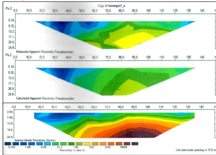
Gambar 6 (a) Penampang Resistivitas untuk Bentangan A Tahun 2012
