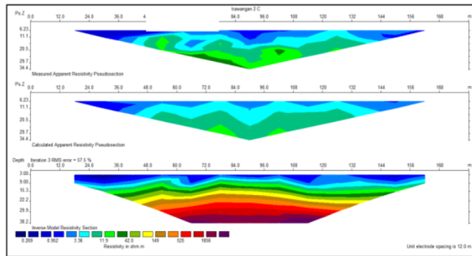
Gambar 7 (b). Penampang Resistivitas untuk Bentangan B Tahun 2014
