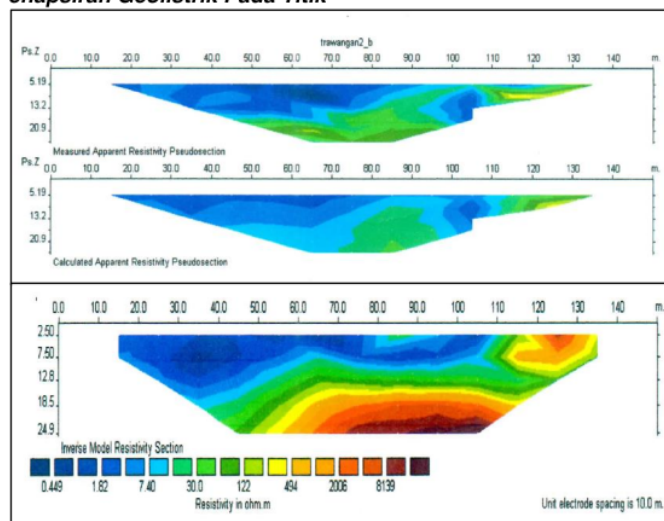
Gambar 7 (a) Penampang Resistivitas untuk Bentangan B Tahun 2012
