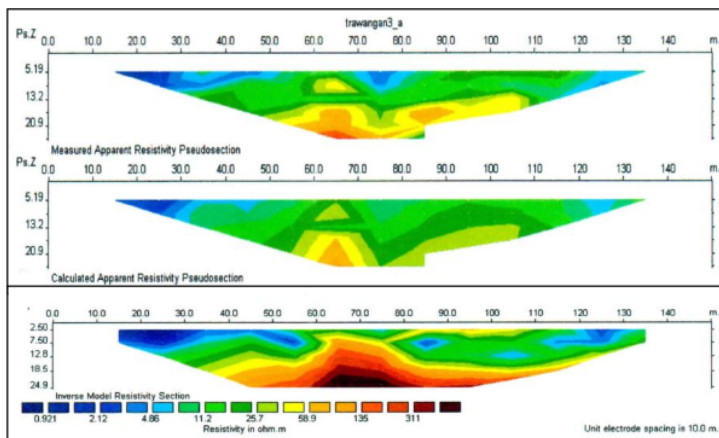
Gambar 8. (a). Penampang Resistivitas untuk Bentangan C Tahun 2012
