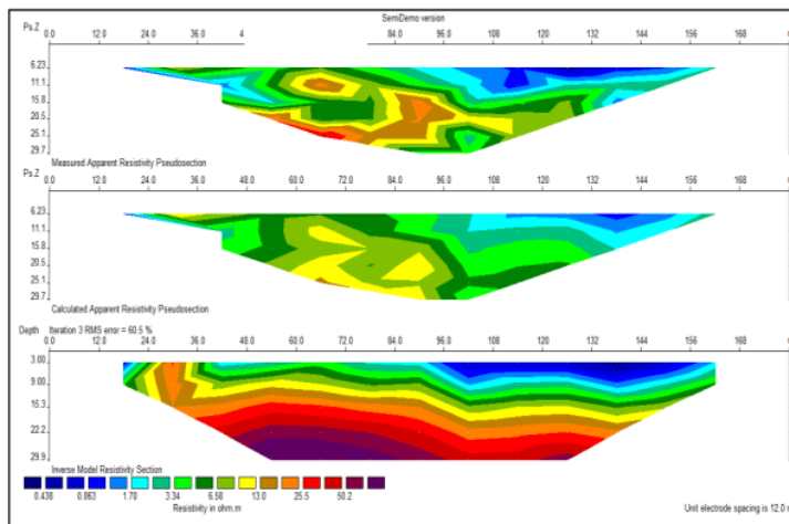
Gambar 8. (b). Penampang Resistivitas untuk Bentangan C Tahun 2014
