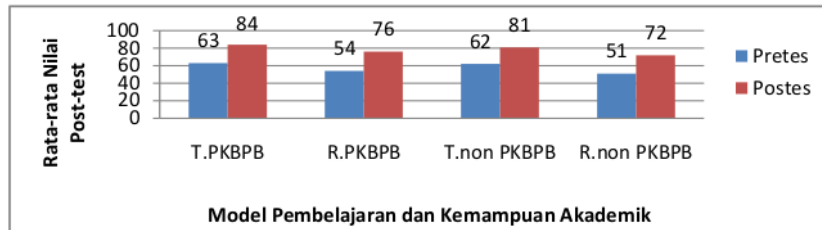
Gambar 2. Rata-rata Nilai Hasil Belajar.
