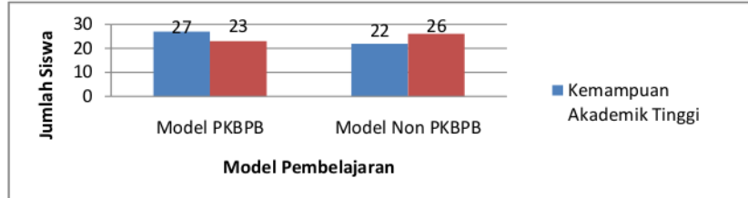
Gambar 1. Sebaran Siswa Berdasarkan Katagori Kemampuan Akademik Siswa.
