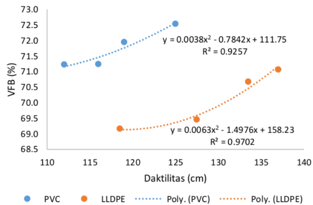
Gambar 3. Hubungan Antara Daktalitas Aspal Modifikasi dan Nilai VFB
