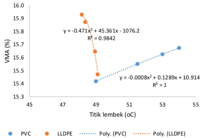
Gambar 7. Hubungan Antara Titik Lembek Aspal Modifikasi dan Nilai VMA
