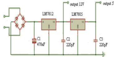
Gambar 7. Rangkaian Catu Daya
