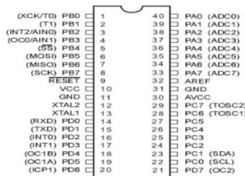
Gambar 2. Konfigurasi Pin Mikrokontroler
