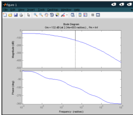
Gambar 16. Respon Frekuensi Sistem Robust pada motor DC 2
