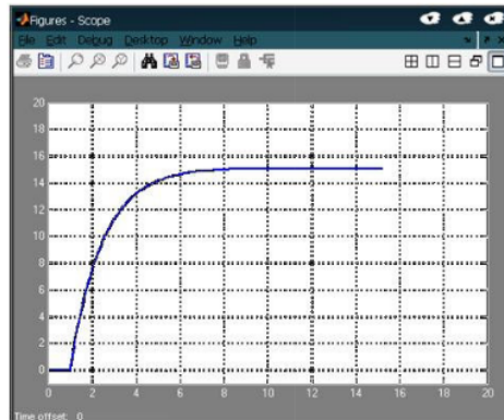
Gambar 12. Grafik hasil respon motor dc 2 pada Matlab
