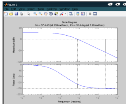
Gambar 15. Respon Frekuensi Sistem Robust pada motor DC 1
