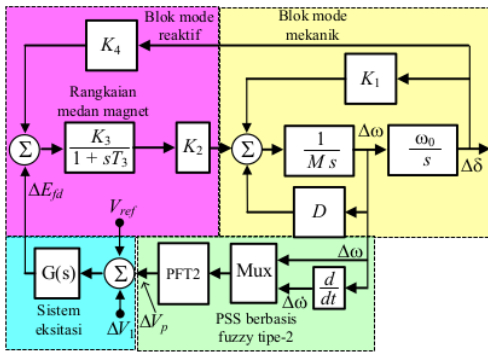
Gambar 2. Diagram blok mesin tunggal dilengkapi dengan PFT2
