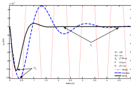
Gambar 11. Perbaikan stabilitas transmisi Tr2 yang dioperasikan
