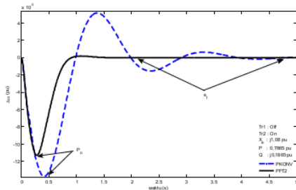
Gambar 12. Perbaikan respons untuk kecepatan rotor
