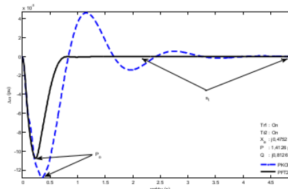
Gambar 18. Perbaikan stabilitas pada beban berat
