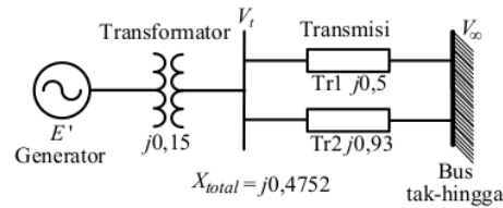
Gambar 16. Reaktansi total untuk transmisi ganda beroperasi
