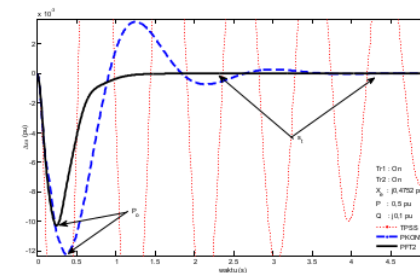
Gambar 17. Unjuk kerja PSS pada beban ringan
