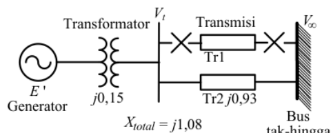
Gambar 10. Rangkaian ekuivalen transmisi ketika TR2 beroperasi
