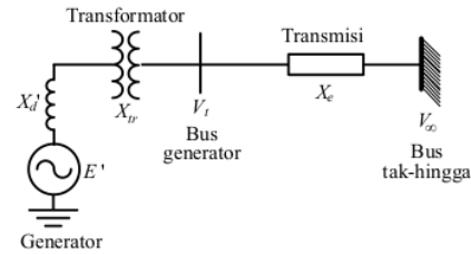
Gambar 1. Diagram segaris mesin tunggal terhubung bus tak-hingga
