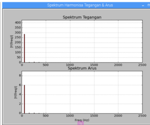
(b) Spektrum tegangan dan arus
