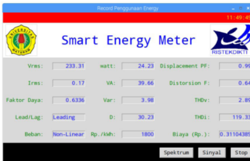
Gambar 15. Hasil rekaman beban charger laptop
