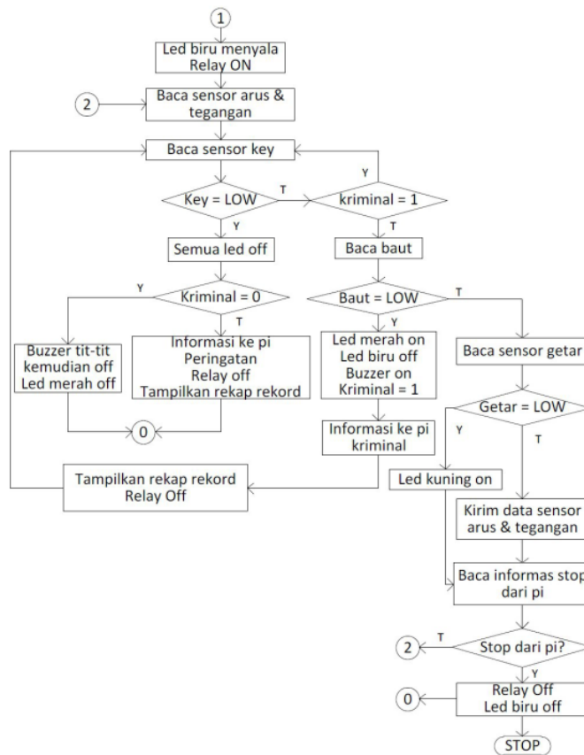
Gambar 5. Diagram alir program pada UNO bagian kedua
