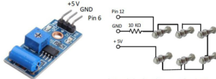
c. Sensor getar SW420 ke pin 6
