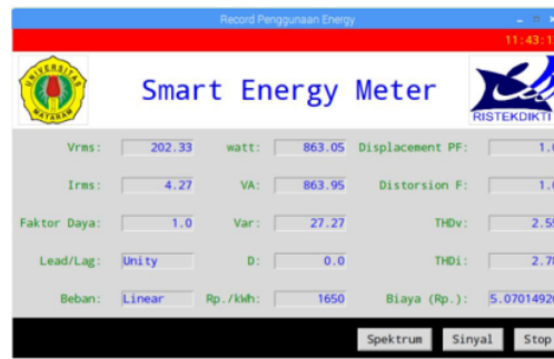
Gambar 11. Hasil rekam SEM untuk beban heater
