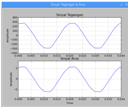
(a) Gelombang tegangan dan arus
