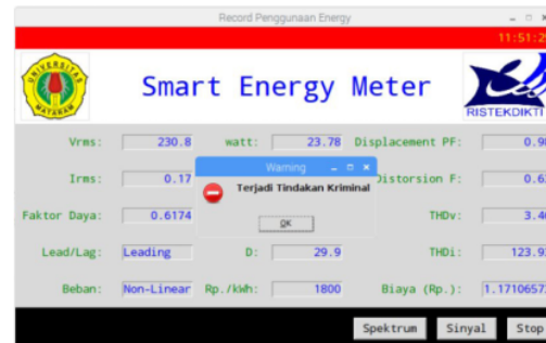
Gambar 8. Baut penutup SEM dibuka saat SEM merekam beban
