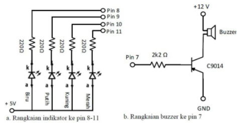
a. Rangkaian indikator ke pin 8-11
