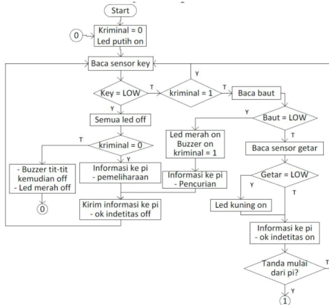
Gambar 4. Diagram alir program pada UNO bagian pertama
