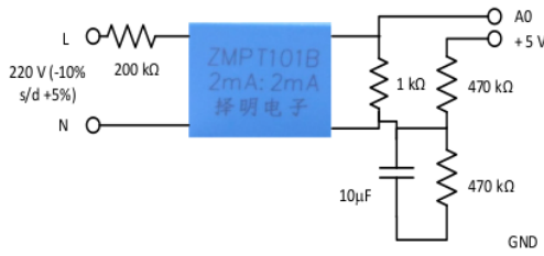
(a). Sensor tegangan
