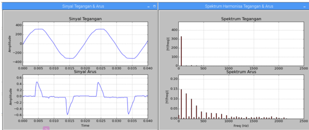
(a) Gelombang tegangan dan arus
