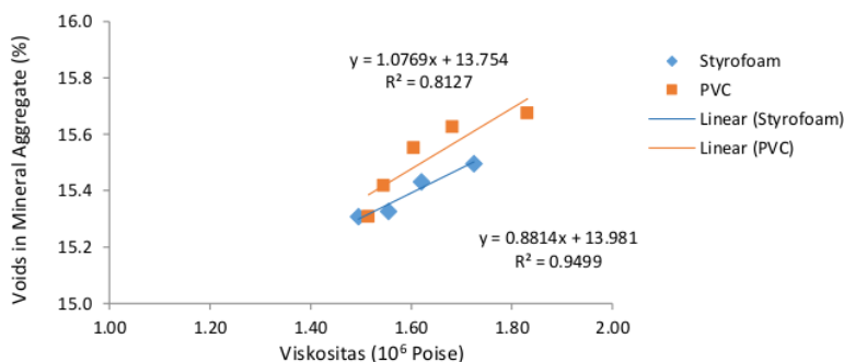
Gambar 1. Grafik hubungan viskositas dan VMA
