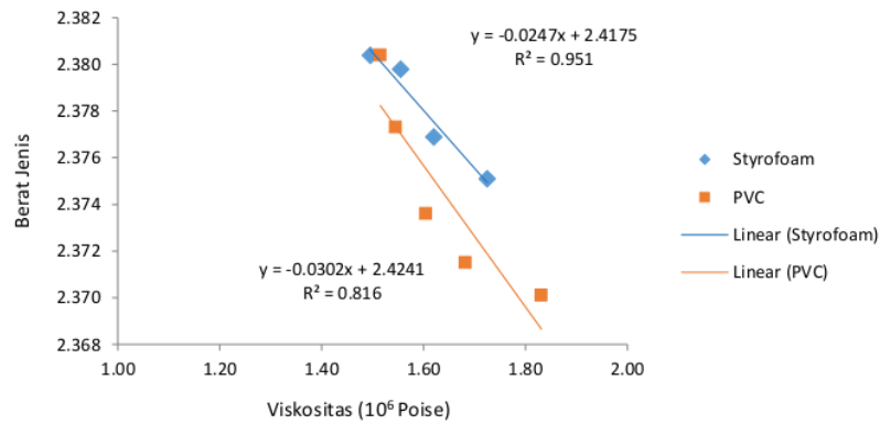
Gambar 4. Grafik hubungan viskositas dan berat jenis
