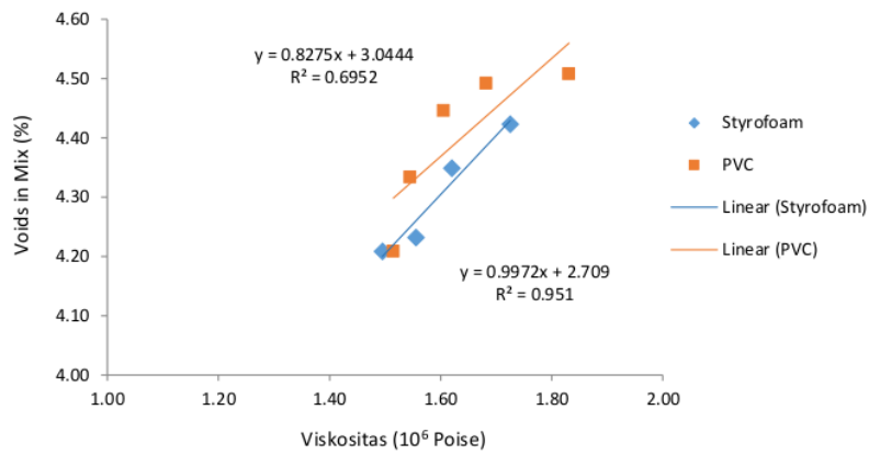
Gambar 2. Grafik hubungan viskositas dan VIM
