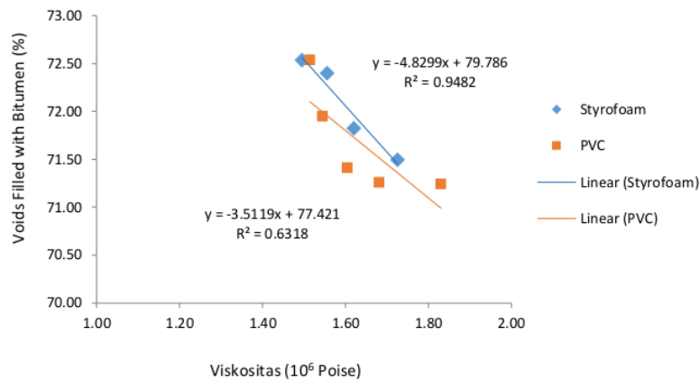
Gambar 3. Grafik hubungan viskositas dan VFB
