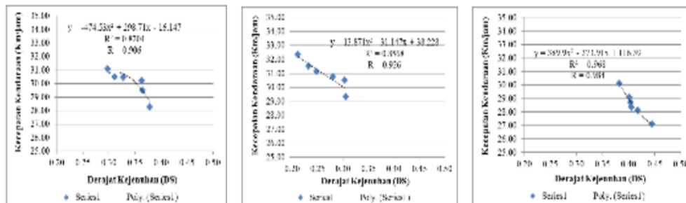
Gambar 6. Grafik hubungan Derajat Kejenuhan dengan Kecepatan Kendaraan Jalan Brawijaya Hari Sabtu, Minggu dan hari Senin
