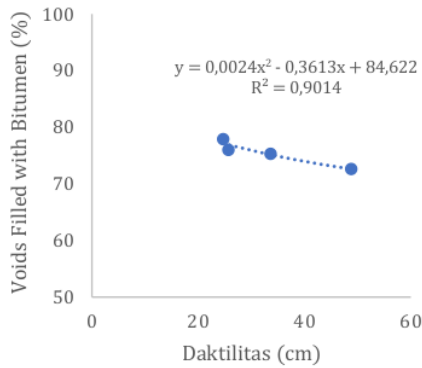
Gambar 3. Grafik hubungan daktilitas dengan nilai VFB
