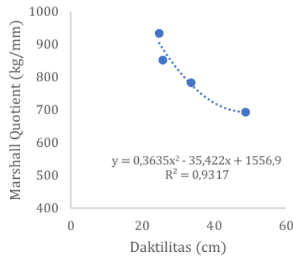
Gambar 6. Grafik hubungan daktilitas dengan Marshall Quotient
