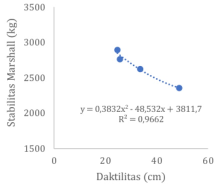
Gambar 4. Grafik hubungan daktilitas dengan stabilitas Marshall campuran
