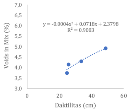
Gambar 1. Grafik hubungan daktilitas dengan nilai VIM
