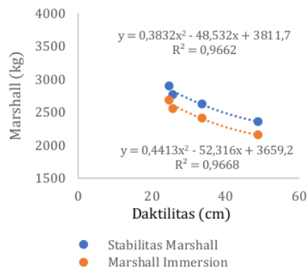
Gambar 7. Grafik hubungan daktilitas dengan nilai Marshall immersion
