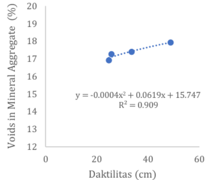
Gambar 2. Grafik hubungan daktilitas dengan nilai VMA
