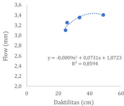
Gambar 5. Grafik hubungan daktilitas dengan nilai flow
