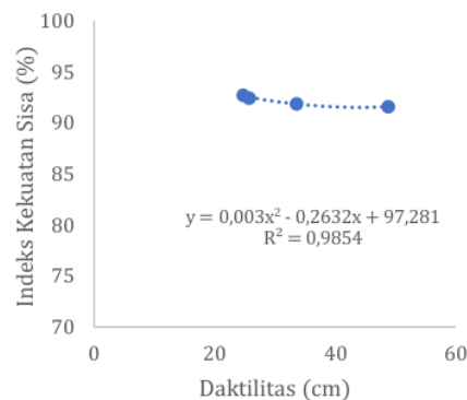
Gambar 8. Grafik hubungan daktilitas dengan nilai IKS
