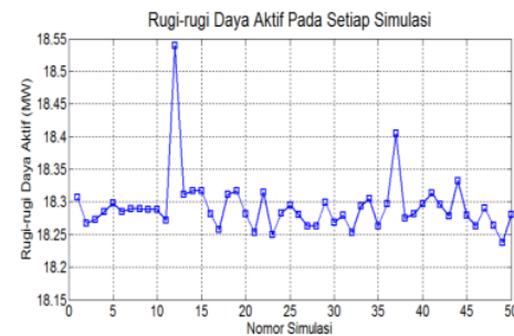
Gambar 6. Rugi-rugi Daya Aktif Pada Setiap Simulasi
