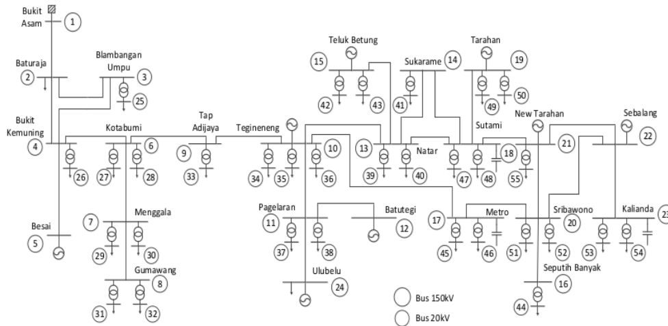
Gambar 4. Diagram Satu Garis Sistem Lampung
