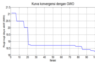
Gambar 3. Kurva Konvergensi Dengan GWO
