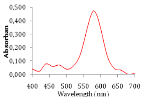
Gambar 2. Spektrum senyawa kompleks Hg-TMK, \lambda_{max} sekitar 574 nm
