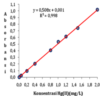
Gambar 5. Kurva linieritas hubungan absorbansi dan konsentrasi Hg(II)
