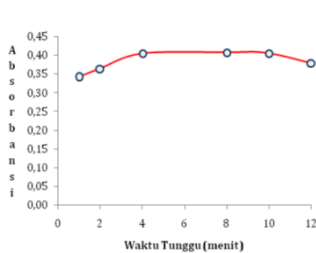
Gambar 4. Kurva hubungan antara absorbansi dan waktu kestabilan
