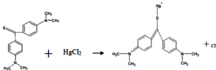
Gambar 1. Reaksi pembentukan senyawa kompleks Hg-TMK
