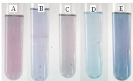
Gambar 1. Beragam produk senyawa kompleks Hg-TMK yang terbentuk: A) kelebihan pereaksi, (B) kelebihan sedikit pereaksi, (C) pH terlalu tinggi, (D) kondisi yang tepat, (E) kondisi adanya ion Ag, Cu, Au, Co, Ni, Fe 1 ppm
