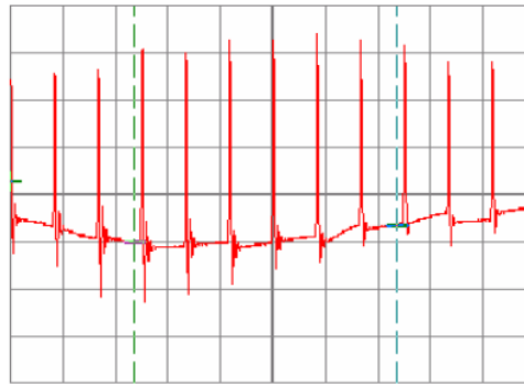
Gambar 9. Lampu TL Philips Life Max 1 pada catu 160 V, frekuensi switching 600 Hz, tanpa kapasitor dan Trafo. Tegangan 100 V/Div, TB 1 ms/Div
