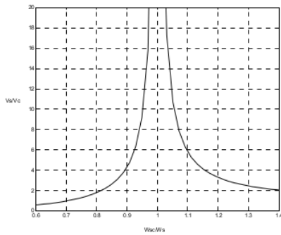
Gambar 1. Grafik perubahan tegangan
