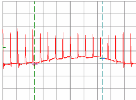
Gambar 10. Lampu TL Philips Life Max 2 pada catu 160 V, frekuensi switching 900 Hz, tanpa kapasitor dan Trafo. Tegangan 100 V/Div, TB 1 ms/Div.
