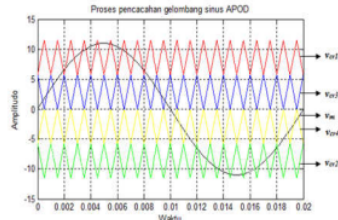
Gambar 3. Teknik Modulasi multicarrier dengan cara menggeser fasa ( level-shifted ) skema APOD
