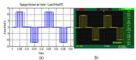
Gambar 17. Tegangan keluaran sel inverter 1 menggunakan skema IPD
