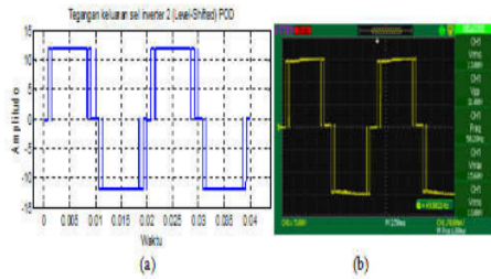
Gambar 21. Tegangan keluaran sel inverter 2 menggunakan skema POD
