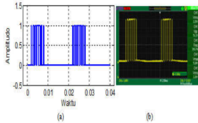
Gambar 12. Bentuk PWM sakelar S_7 skema APOD
