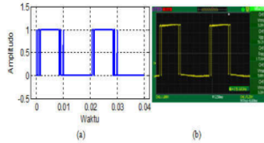
Gambar 11. Bentuk PWM sakelar S_5 skema POD
