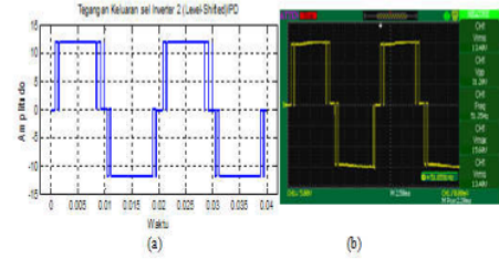
Gambar 18. Tegangan keluaran sel inverter 2 menggunakan skema IPD
