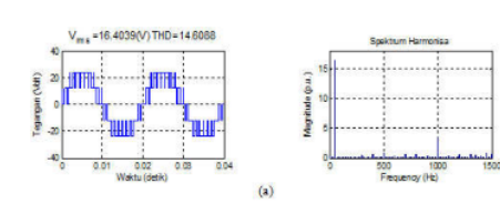
Gambar 18. Tegangan keluaran sel inverter 2 menggunakan skema IPD
