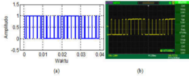
Gambar 6. Bentuk PWM sakelar S_1 modulasi phase-shifted
