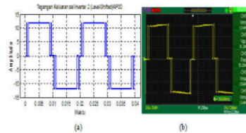
Gambar 24 Tegangan keluaran sel inverter 2 menggunakan skema APOD
