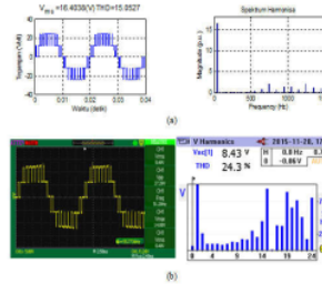
Gambar 25 Tegangan keluaran serta spektrum harmonisa pada inverter menggunakan teknik modulasi multicarrier level-shifted skema APOD
