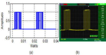
Gambar 10. Bentuk PWM sakelar S_7 skema POD
