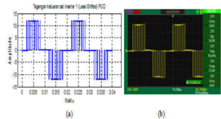
Gambar 20. Tegangan keluaran sel inverter 1 menggunakan skema POD
