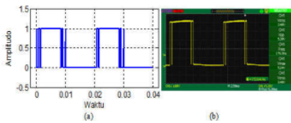
Gambar 9. Bentuk PWM sakelar S_5 skema IPD
