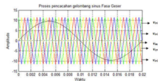
Gambar 1. Teknik Modulasi multicarrier dengan ara menggeser fasa ( phase-shifted )
