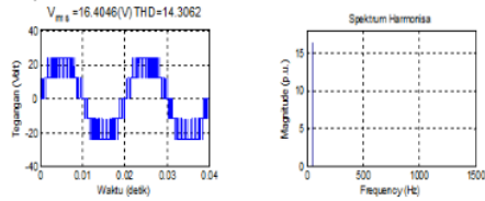
Gambar 15. Tegangan keluaran sel inverter 2 menggunakan teknik modulasi multicarrier phase-shifted
