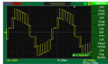
Gambar 30. Tegangan keluaran inverter multilevel Cascaded H-Bridge (CHB) dengan teknik modulasi multicarrier Level-Shifted skema POD
