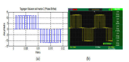
Gambar 15. Tegangan keluaran sel inverter 2 menggunakan teknik modulasi multicarrier phase-shifted
