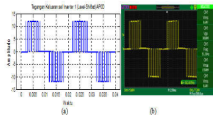
Gambar 23. Tegangan keluaran sel inverter 1 menggunakan skema APOD
