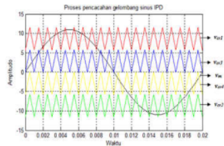
Gambar 2. Teknik Modulasi multicarrier dengan cara menggeser fasa ( level-shifted ) skema IPD
