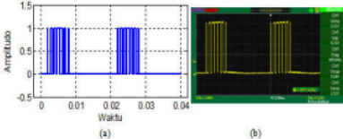
Gambar 8. Bentuk PWM sakelar S_1 skema IPD
