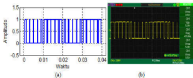
Gambar 7. Bentuk PWM sakelar S_3 modulasi phase-shifted
