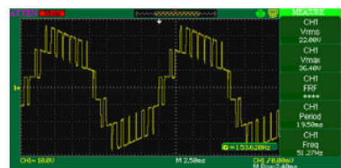
Gambar 31. Tegangan keluaran inverter Multilevel Cascaded H-Bridge (CHB) dengan teknik modulasi multicarrier Level-Shifted skema APDO
