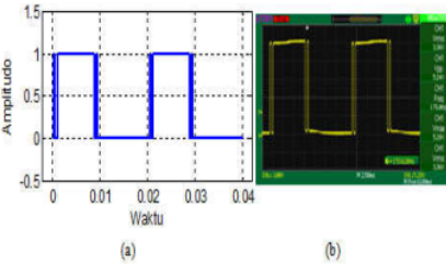
Gambar 13. Bentuk PWM sakelar S_5 skema APOD
