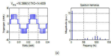
Gambar 21. Tegangan keluaran sel inverter 2 menggunakan skema POD
