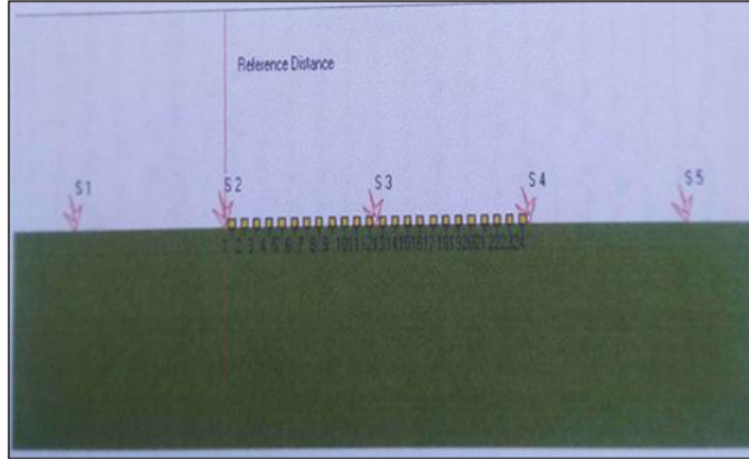
Gambar 3. Skema Lintasan dan Pemasangan Geophone
