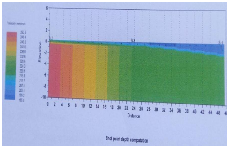
Gambar 7. Penampang 2D Lapisan Bawah Permukaan
