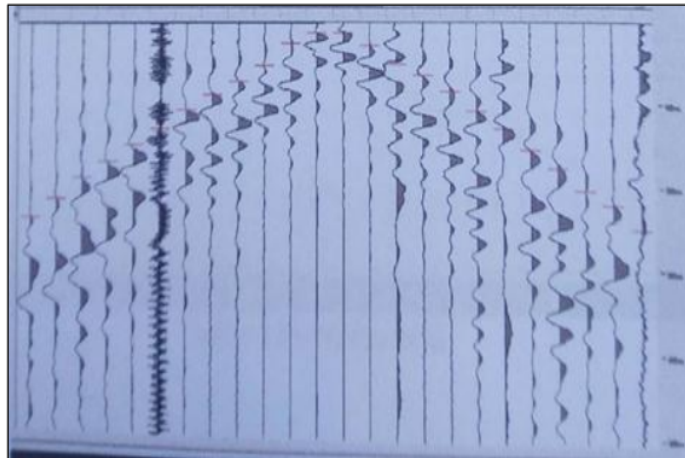
Gambar 4. Proses Picking Data Seismik Refraksi
