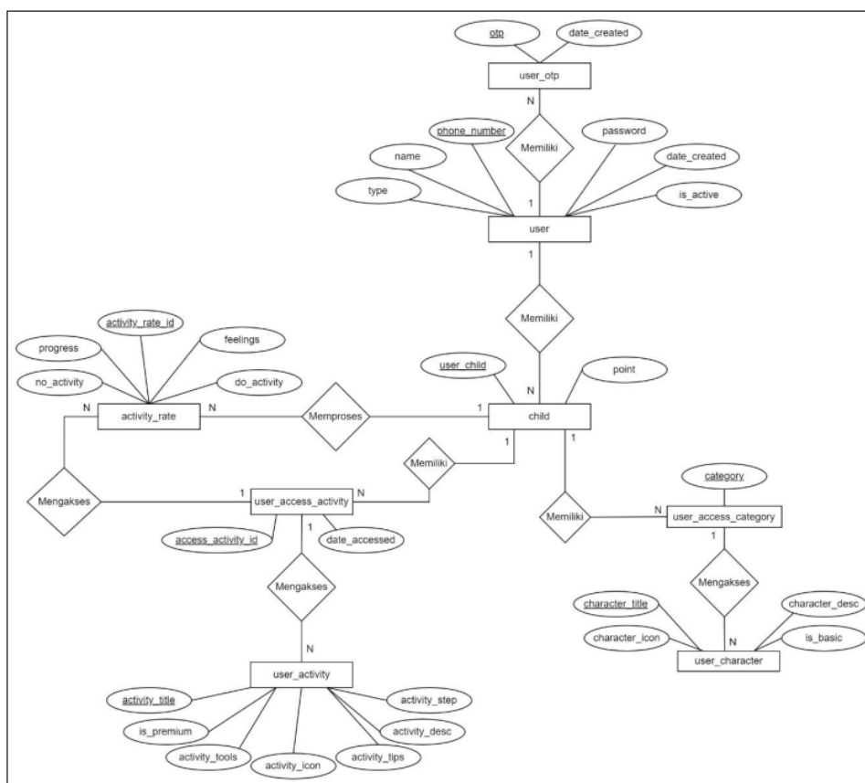
Gambar 4. ERD Sistem Informasi Parenting
