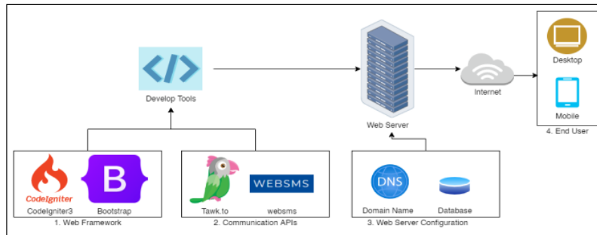
Gambar 5. Arsitektur sistem
