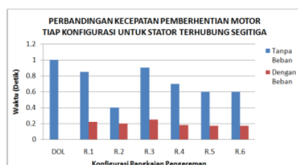
Gambar 18. Grafik perbandingan kecepatan pemberhentian motor tiap konfigurasi untuk stator terhubung segitiga
