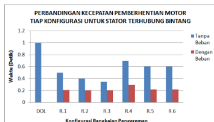
Gambar 17. Grafik perbandingan kecepatan pemberhentian motor tiap konfigurasi untuk stator terhubung bintang
