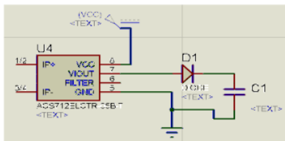
Gambar 8. Rangkaian Sensor Arus
