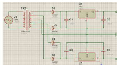
Gambar 6. Rangkaian Catu Daya
