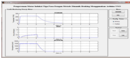
Gambar 16. Pengujian metode Direct On-Line (DOL) konfigurasi bintang
