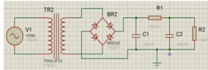
Gambar 9. Rangkaian Sensor Tegangan
