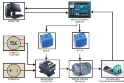
Gambar 5. Blok Diagram Rancangan Sistem
