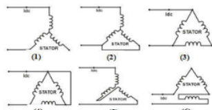
Gambar 3. Konfigurasi rangkaian stator (Warsito, 2006)
