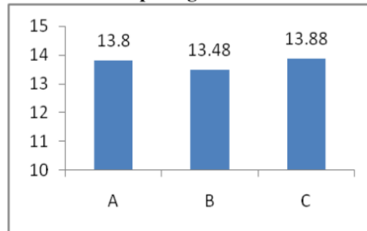
Gambar 1. Kadar air kering udara papan laminasi bambu petung
