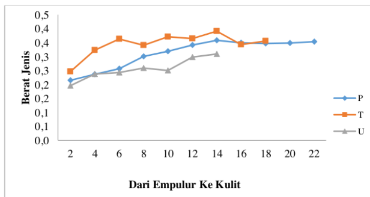
Gambar 5. Grafik Pola Berat Jenis Kering Tanur Dari Dekat Empulur
