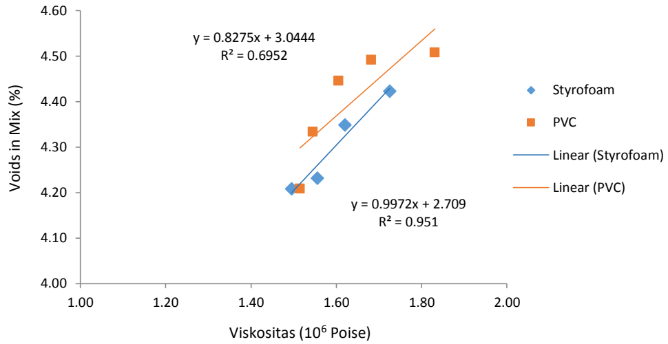
Gambar 2. Grafik hubungan viskositas dan VIM
