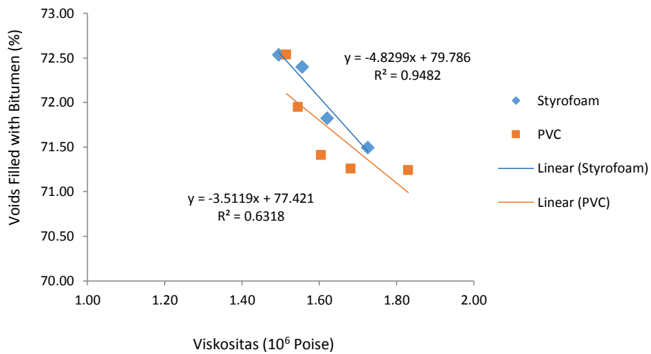
Gambar 3. Grafik hubungan viskositas dan VFB
