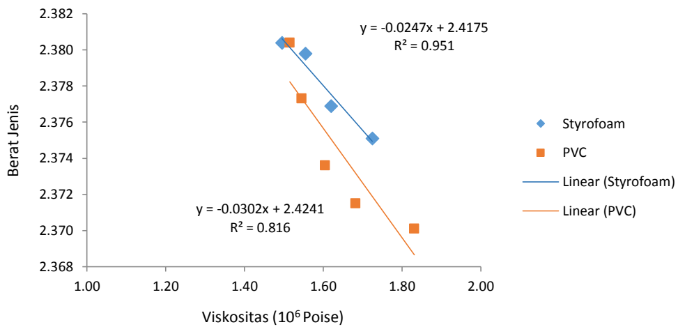
Gambar 4. Grafik hubungan viskositas dan berat jenis
