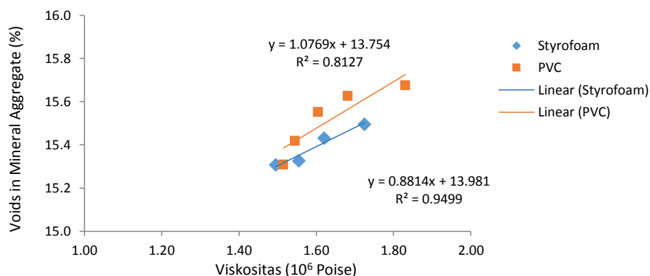
Gambar 1. Grafik hubungan viskositas dan VMA
